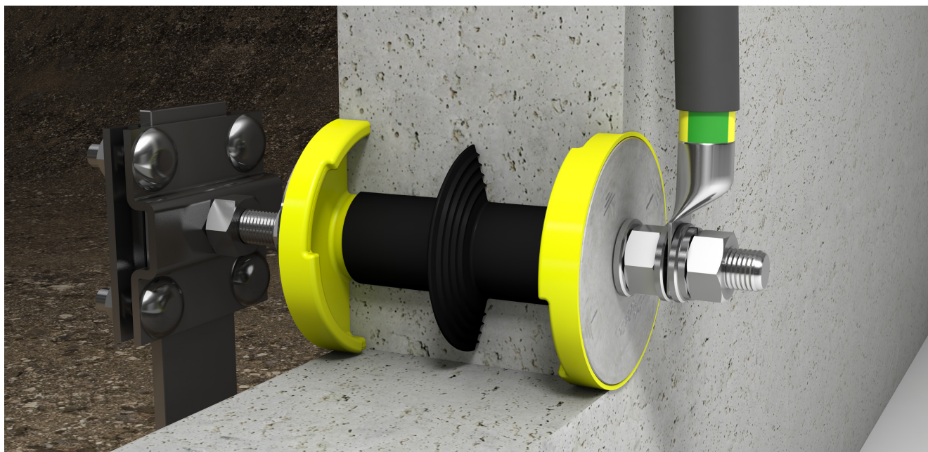
Passage de mise à la terre HEA-IS-M12: d'un côté, raccordement à barre d'acier plat par borne de fixation en croix Z-KG-M12 et de l'autre côté, raccordement d'un conducteur de terre par boulon de raccord Z-B-M12.
