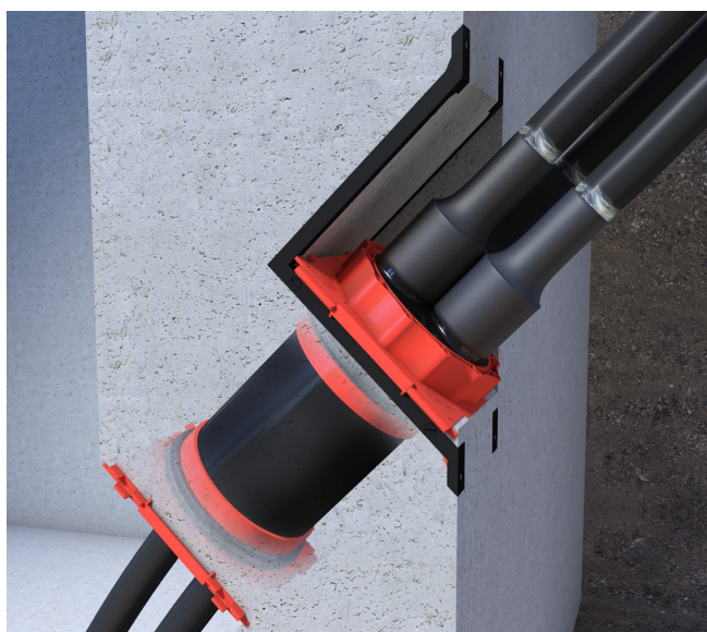
Fourreau oblique étanche HSI 150-K2 S45°/X et couvercle HSI 150-D3/58
